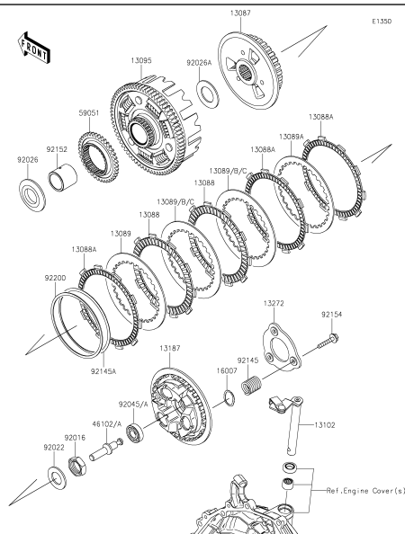
10 Clutch
