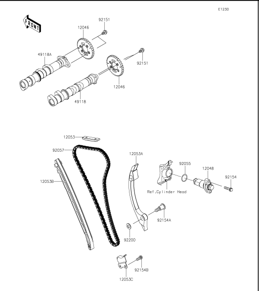
7 Camshaft(s)/Tensioner
