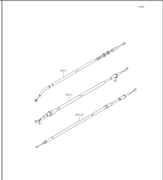
52 Cables
