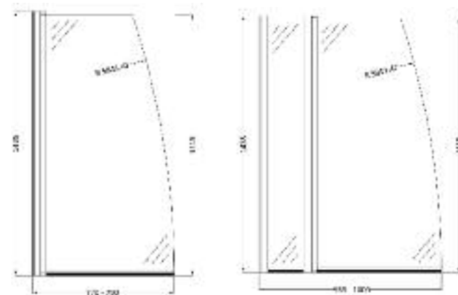
NSS1-NSSS2-NSSSR1-NSSSR2 SAIL BATH SCREENS
