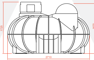
END ELEVATION
