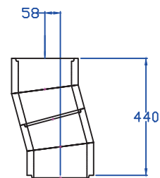
OFFSET DIMENSIONS PER PAIR
